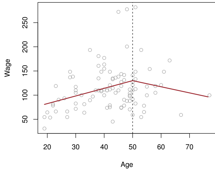
Linear Spline
